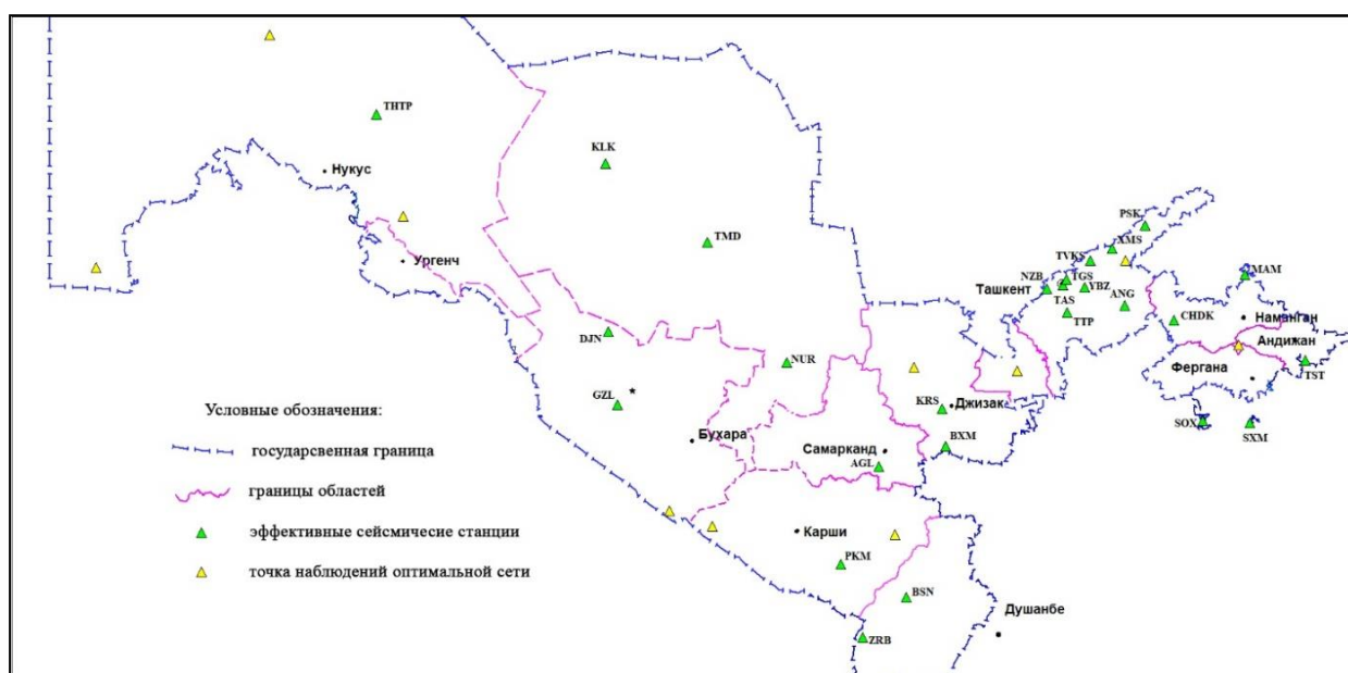
Рисунок 5. Оптимальная сеть сейсмических наблюдений
