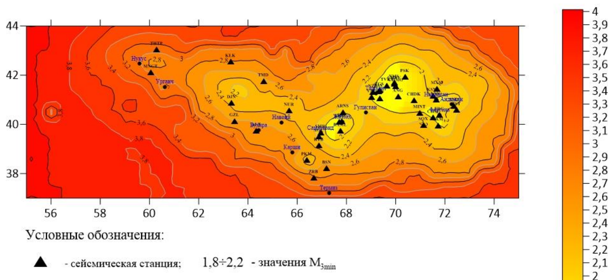
Рисунок 2. Схематическая карта представительности M_{3min} регистрации землетрясений (по данным сети РЦСМ МЧС на 2020 г.)
