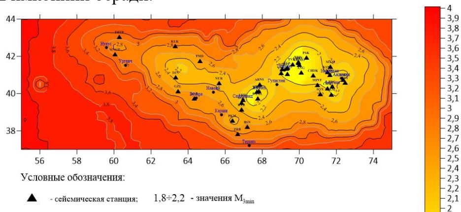
2-расм. Зилзилаларни қайд этишнинг қуйи чегарасини M_{3min} схематик харитаси (ФВВ СМРМ тармоғи бўйича 2020 й)
