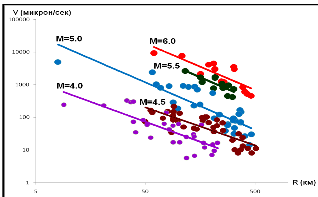
1-расм. Фарғона ботиклигида магнитудаси M=4,0-6,0 бўлган зилзилалар учун грунтнинг тебраниш тезлиги амлитудалари сўнишининг экспериментал маълумотлари
