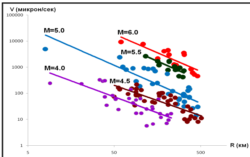
Рисунок 1. Экспериментальные данные затухания амплитуд скоростей колебаний грунта при землетрясениях с магнитудой M=4-6 в Ферганской межгорной впадине
